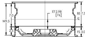
SECTION D-D
